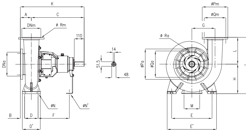
DN = Brida UNI EN 1092-1 PN16 – Cotas aproximadas
